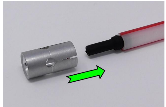
1.4 WGT über den Blindstopfen fädeln und auf das Mikrorohr aufdrücken.
